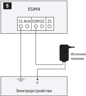
Схема подключения входа
